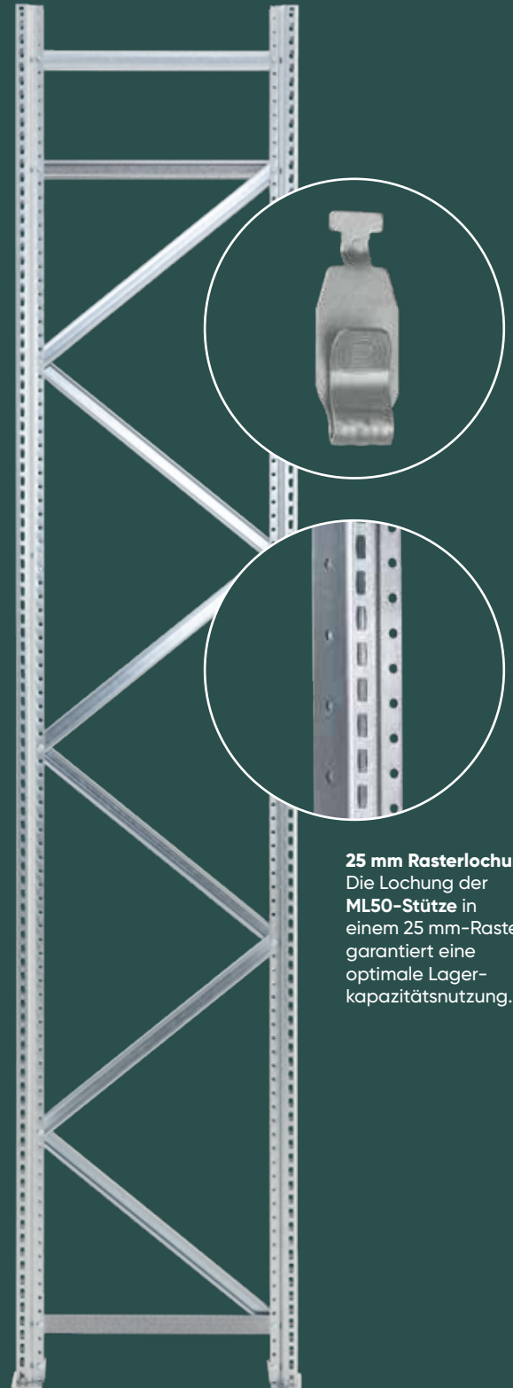
↑ MULTILOAD ML50-Rahmen
