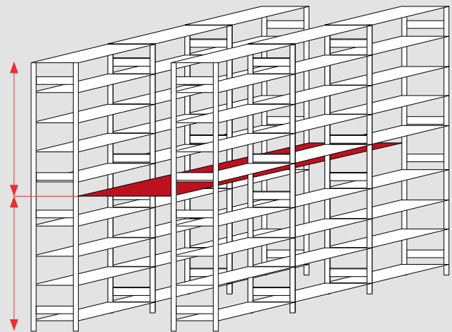
2 -geschossige Fachbodenregalanlage
