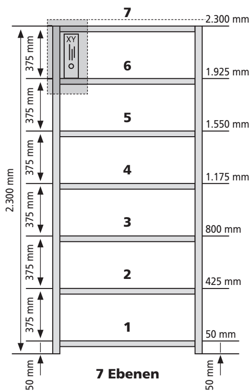
Regalhöhe 2.300 mm
